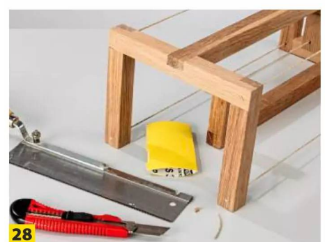
28 Sind alle fünf Schnüre gespannt, schneiden Sie die Schnur- und Dübelenden bündig zum Holzgestell ab.
