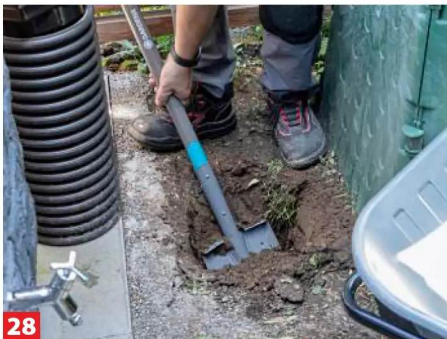
28 Ohne Kanalanschluss ist ein Versickerungsschacht praktisch. Dafür eine 50 x 50 x 70 cm große Grube ausheben.
