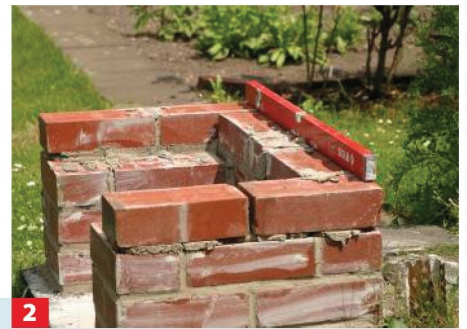
2 Mauern Sie stets im Versatz (hier: Halbsteinverband), legen Sie gleichmäßig dicke Mörtelfugen an und richten jede Lage darin aus.
