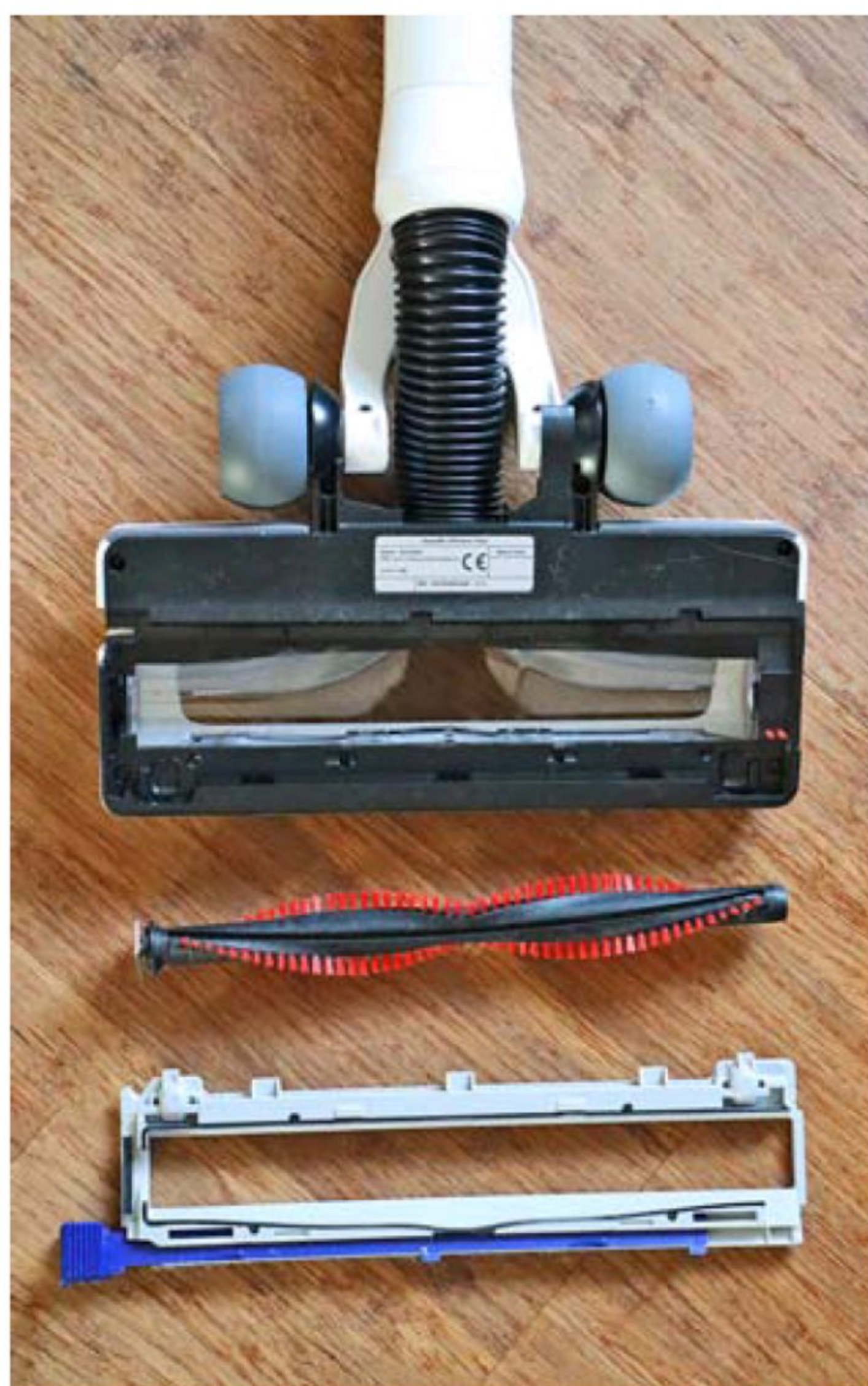
WARTUNGSFREUNDLICH: Ob Entfernen von aufgewickelten Haaren oder Tausch der Bürste: Alles gelingt werkzeuglos und spielend einfach.
