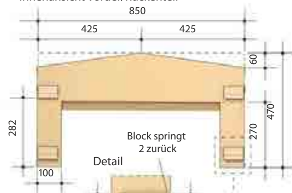
Innenansicht Vorder/Rückenteil
