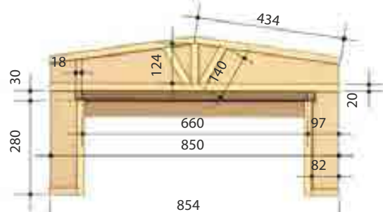
Innenansicht Vorder/Rückenteil
