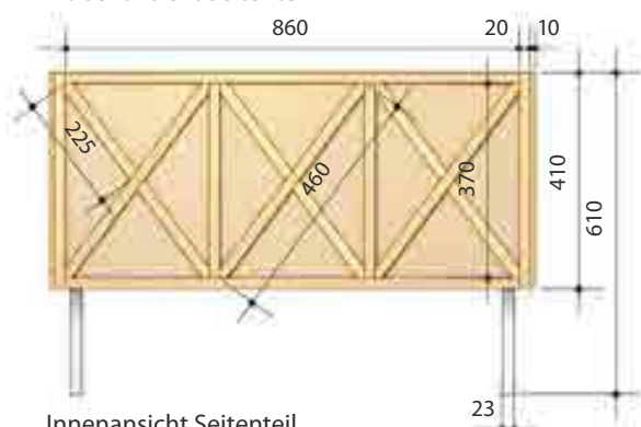
Innenansicht Seitenteil
