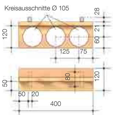
Ansichten Topfhalter
