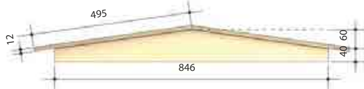
Vorderansicht Dach
