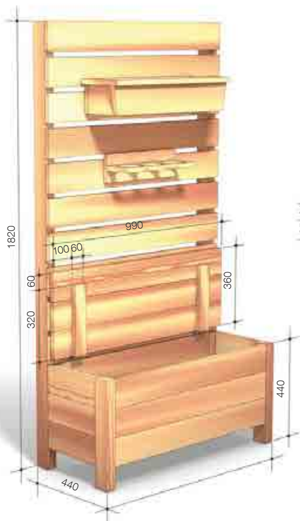
Ansichten Kübelhalter
