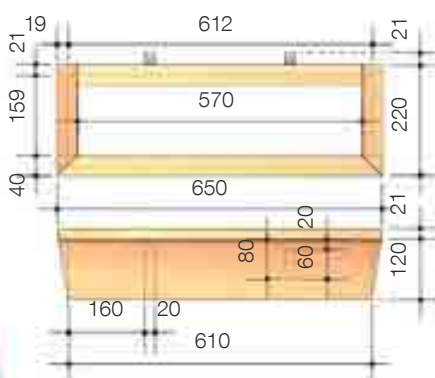
Ansichten Kübelhalter
