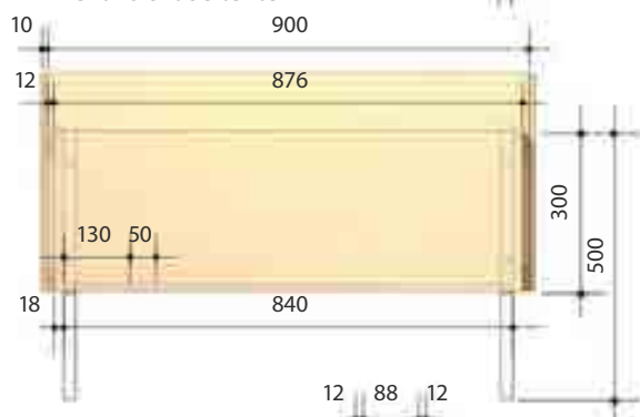
Schnitt
