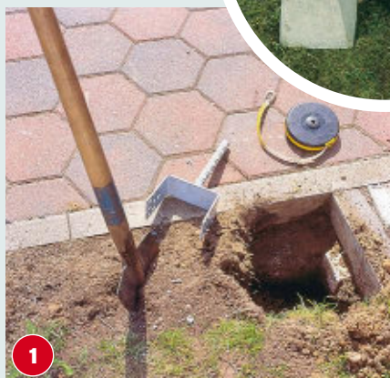
Prüfen, ob betonierte Wegkanten die Arbeit stören. Danach die Löcher für das Fundament graben.
