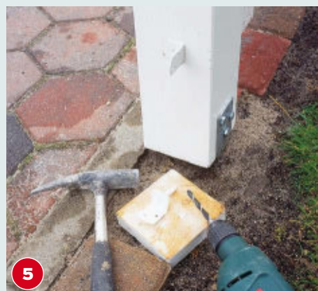
Löcher für die L-Beschläge vorbohren. Mit leichten Hammerschlägen etwa 1 cm tief einschlagen und dann eindrehen.
