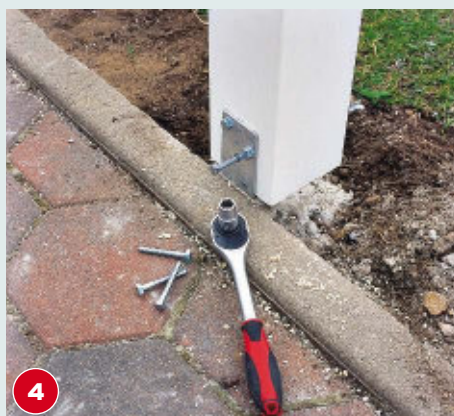
Eine Knarre mit Stecknuss ist ein Segen, wenn insgesamt sechs Schrauben je Pfosten eingeschraubt werden müssen.
