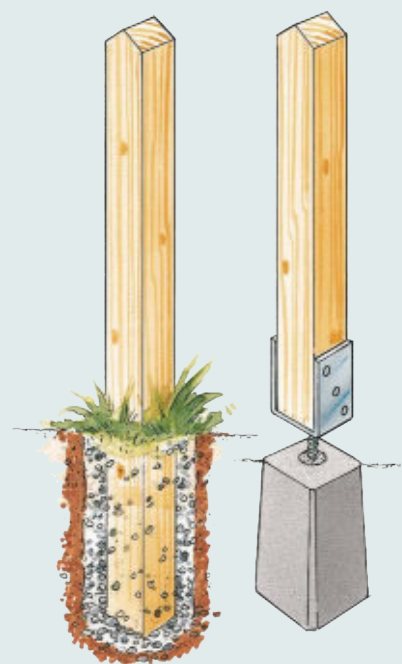
Pfosten direkt einzugraben, macht sie anfällig für Nässe. Besser: Pfostenschuhe nehmen
