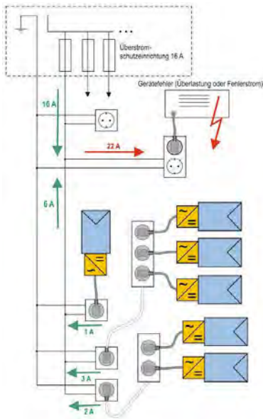
Der Stromanteil , der von den Modulen in den Endstromkreis eingespeist wird, wird von der Überstromschutzeinrichtung nicht erfasst.
