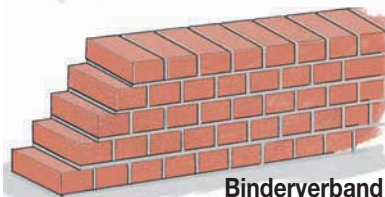
Binderverband
