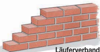
Läuferverband
