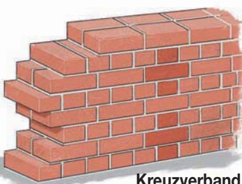
Kreuzverband
