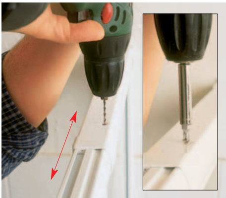
13 Die in Länge und Winkel ausgerichteten Querträgerprofile werden von oben vorgebohrt und anschließend mit Schrauben festgesetzt.
