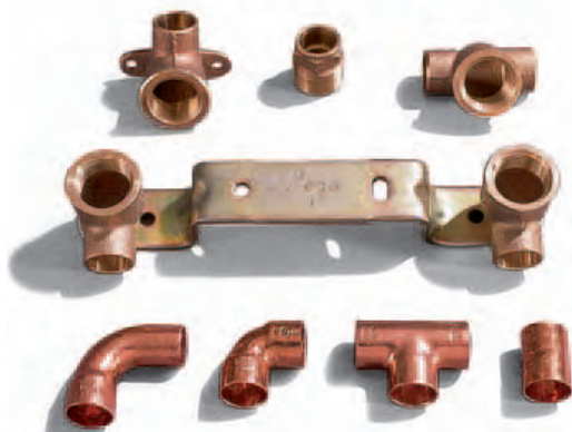
Die Fittings sind die verbindenden Teile: Bögen, T-Stücke, Muffen, Übergänge und Wandscheiben werden mit dem Rohr verlötet.
