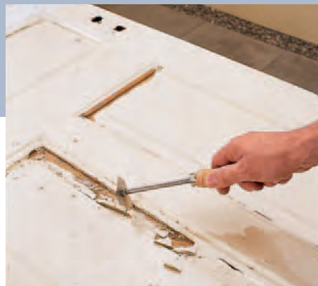
4 Mit dem Dreikantschaber können die losen und hochgekommenen Lackstellen und Blasen an den Profilen der Tür herausgekratzt werden.
