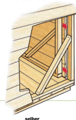
Elementbauweise
