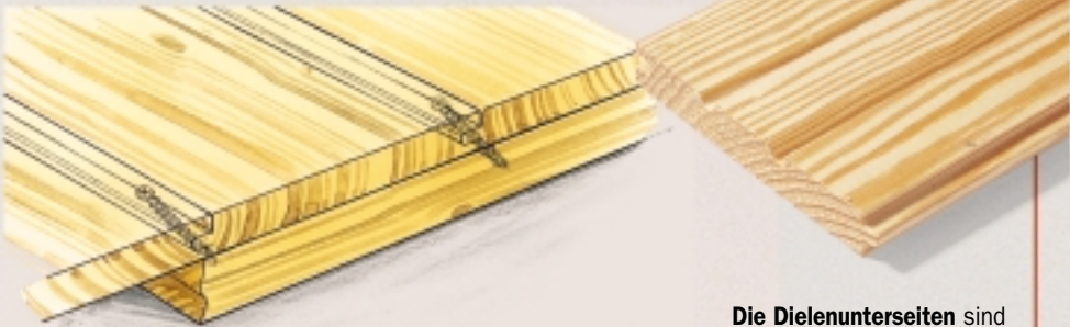
Die Dielenunterseiten sind zweifach genutet („Schwindnuten“), um das Arbeiten des Holzes zu minimieren.
