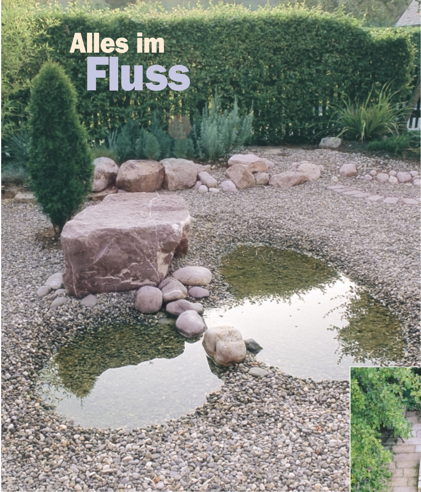
Die Teichfolie liegt auch dort, wo es normalerweise trocken ist. Praktisch ist es, unter der gesamten Kiesfläche Geovlies zu verlegen und im nassen Bereich Folie aufzulegen. Wird die wiederum mit Vlies abgedeckt, schont das die Folie und gibt den Steinen besseren Halt.
