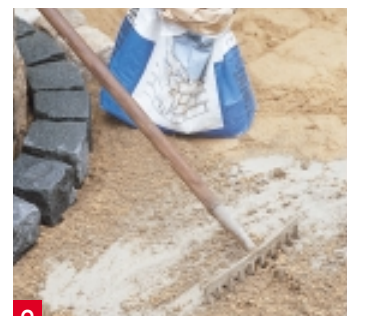
2 Bevor Sie die Granitbossen verlegen, mischen Sie noch Zement unter den Sand. Achten Sie darauf, dass das Gefälle bestehen bleibt.
