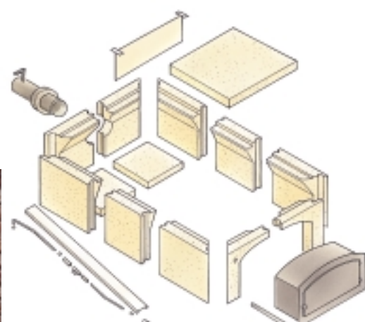
Geschützter Winkel mit Backofen
