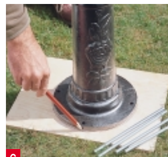
6 Ein Stück Sperrholz dient als Schablone für den Brunnenfuß. Zeichnen Sie Umriss und die Bohrungen für die Gewindestangen auf.
