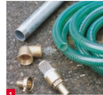
1 Schlauch und Rohr verbinden Sie per 90°-Fitting und Schraubkupplung. Das Saugventil am anderen Schlauchende montieren.
