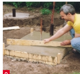
3 Ist der Beton verfüllt , ziehen Sie ihn über den Schalungsrand mit einem geraden Brett ab. Die Oberfläche soll blasenfrei sein.
