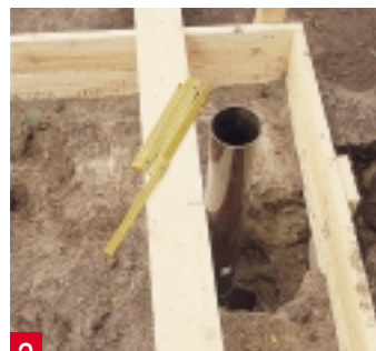
2 Innerhalb der Fundamentschalung graben Sie das Loch für den Zulauf. Ein Kunststoffrohr dient als Schalung für die Betonaussparung.
