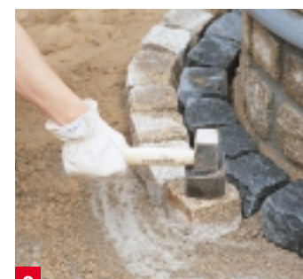
3 Ausgehend vom Betonring legen Sie die Steine. Verwenden Sie zum Festklopfen den schweren Fäustel mit einer Gummi-Schutzkappe.
