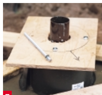
7 Die Schablone legen Sie auf den Sockel und stecken die Gewindestangen durch die Löcher in den frischen Beton. Der Pfeil zeigt nach vorn.
