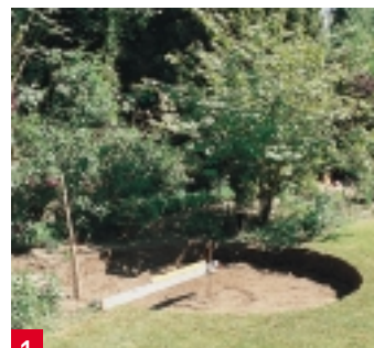
1 Das Erdloch heben Sie 40 cm tief mit der Schaufel aus. Markieren Sie den Mittelpunkt per Pflock, daran zeichnen Sie die Randhöhe an.
