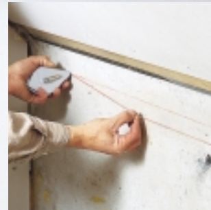
Mit einer Schlagschnur wird zunächst die Montagehöhe für justierbare Profilhalter markiert, die mit 50 cm Abstand (Achismaß) am Drempe montiert werden.
