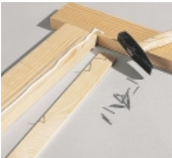
Als Auflage für die Dreieckleisten leimen Sie eine Flachleiste mit 1 cm Überstand rückseitig an die Querhölzer des Rahmens. Zusätzlich fixieren Drahtstifte die Leiste.
