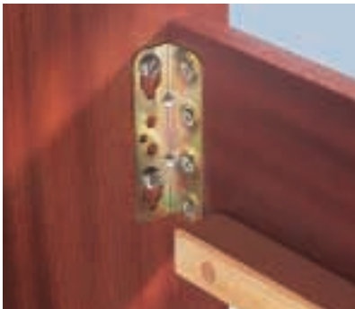
Der Universal-Bettbeschlag ist für die linke wie für die rechte Bettseite geeignet. Er wird über Schrauben mit entsprechend großem Kopf geschoben. (Hettich)
