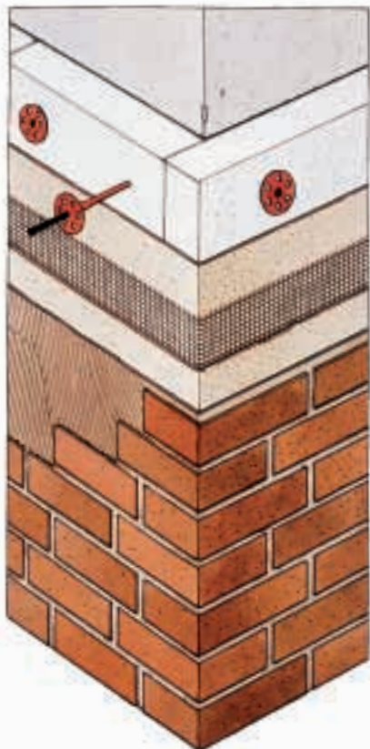
Systematischer Aufbau einer Verblendung mit Wärmedämmung: Dämmplatten, Kleberschicht, Glasfaserarmierung, Kleber und Verblender (von innen nach außen).
