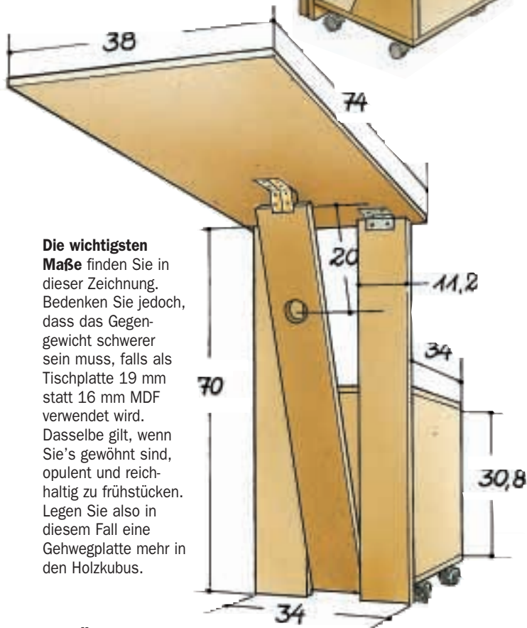
5 Die Rückwand des Tisches wird kopfstehend mit Scharnieren an der klappbaren Tischplatte verschraubt. Achten Sie auf die rechten Winkel!
