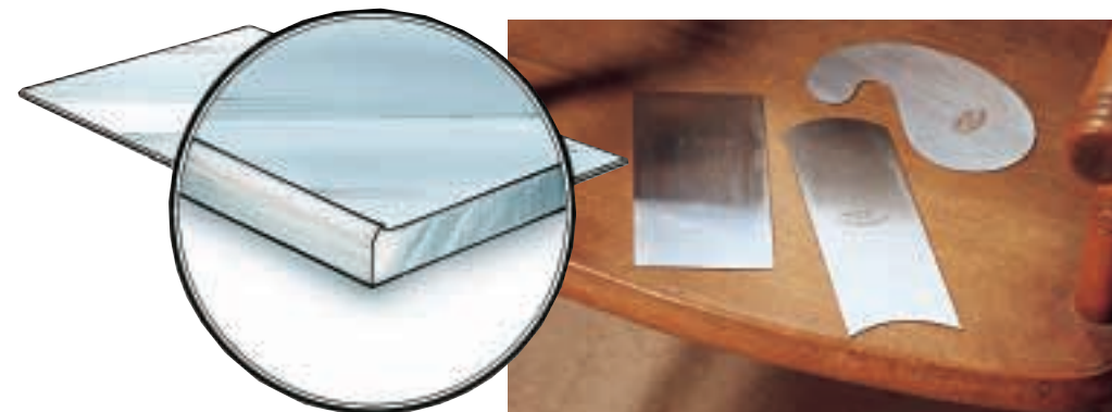
Schwanenhals nennt sich das oval geschwungene Metallblatt. Es ist, wie die anderen Blätter eine Ziehklinge, mit denen besonders feine Holzoberflächen erzielt werden. Geschabt wird mit dem feinen Grat, der mit einer Feile an die Kante gezogen wird.
