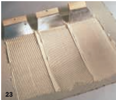
23 Der Teppichkleber wird mit einem Zahnpachtel aufgetragen. Welche der drei Zahnungsgrößen für Belag und Kleber die Richtige ist, steht auf dem Klebergebinde.
