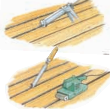
Parkett im Fischgrätmuster Der Holzkitt wird diagonal in die Fugen eingearbeitet.
