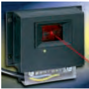
Der Strahl eines Laserpointers auf den Sensor gerichtet, betätigt diesen Schalter. Zielhilfe leistet eine Leuchtdiode. Leistung: 3000 W. (Conrad)
