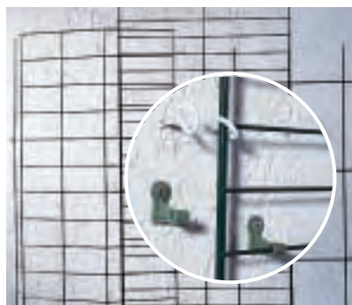
Rankgitter in Trapezform (links), daneben ein leichtes Rankgitter und eine schwere Gitterstabmatte. Zum Befestigen Kunststoff-Wandclips und Hakenschrauben.
