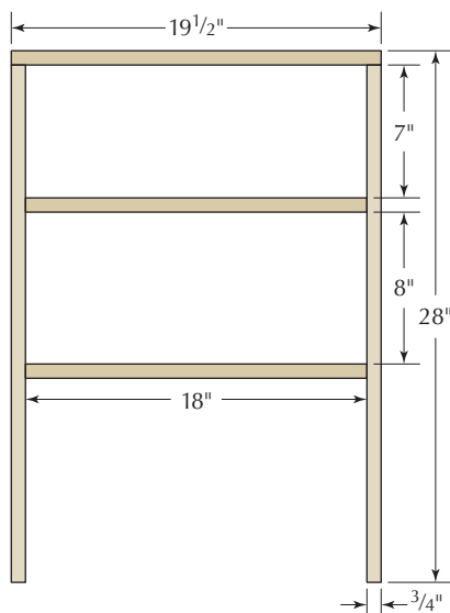
ELEVATION
