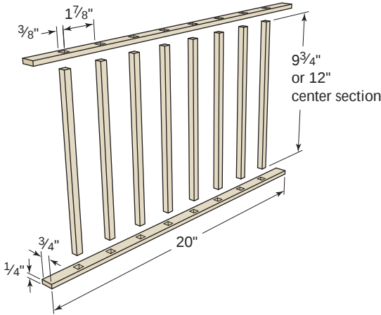
DIVIDER SUBASSEMBLY
