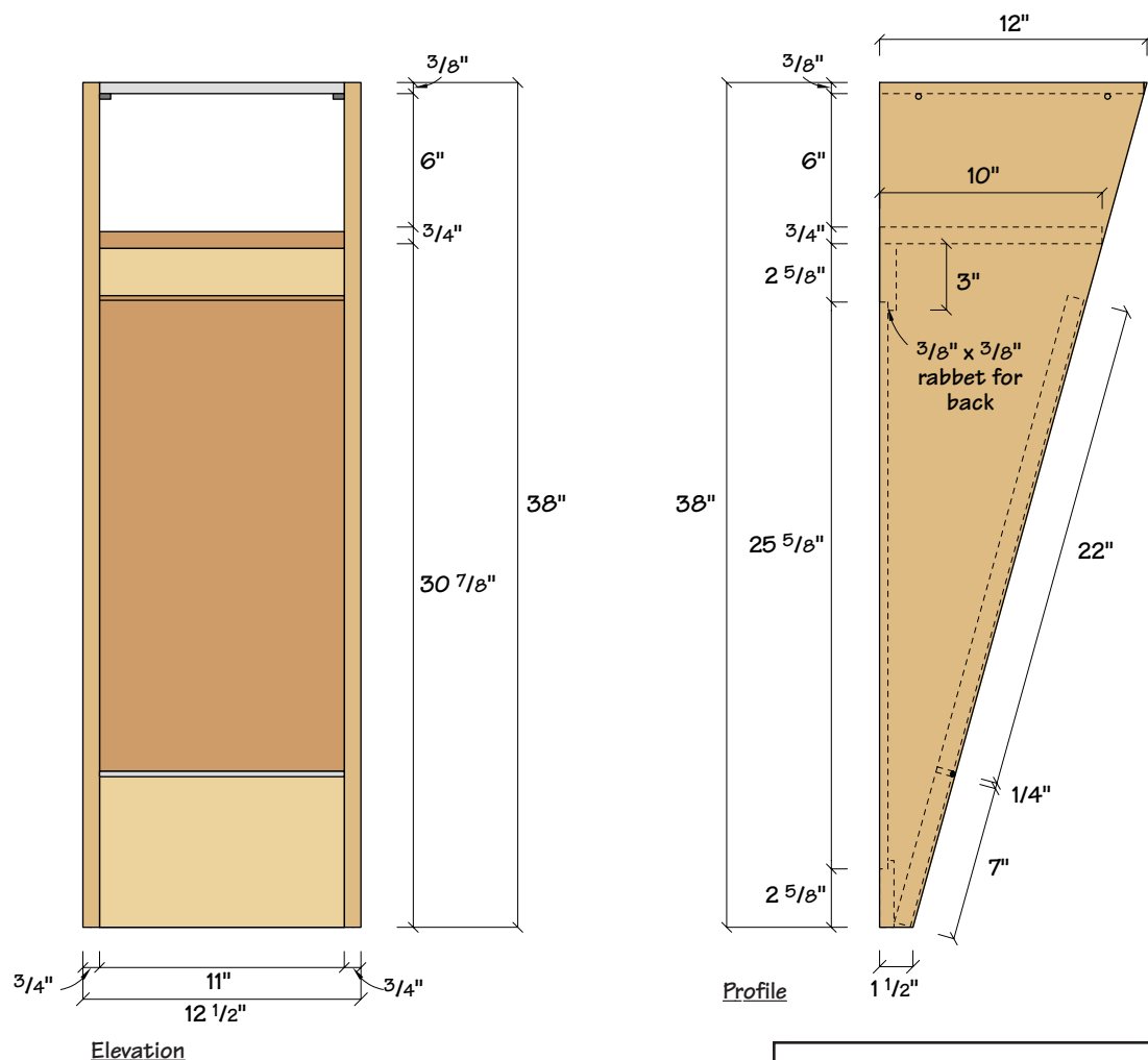
Elevation
