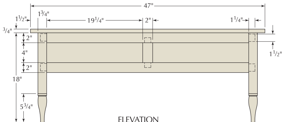
ELEVATION
