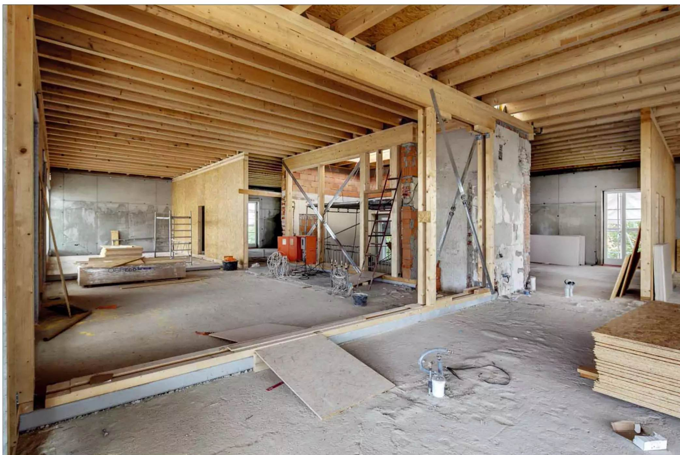
Hier sieht man eine Baustelle, auf der die Unterkonstruktion hauptsächlich aus Holz besteht
