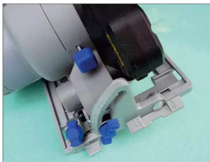
Die meisten Einstellungen werden wie an normalen Handkreissägen vorn am Sägeschuh vorgenommen
