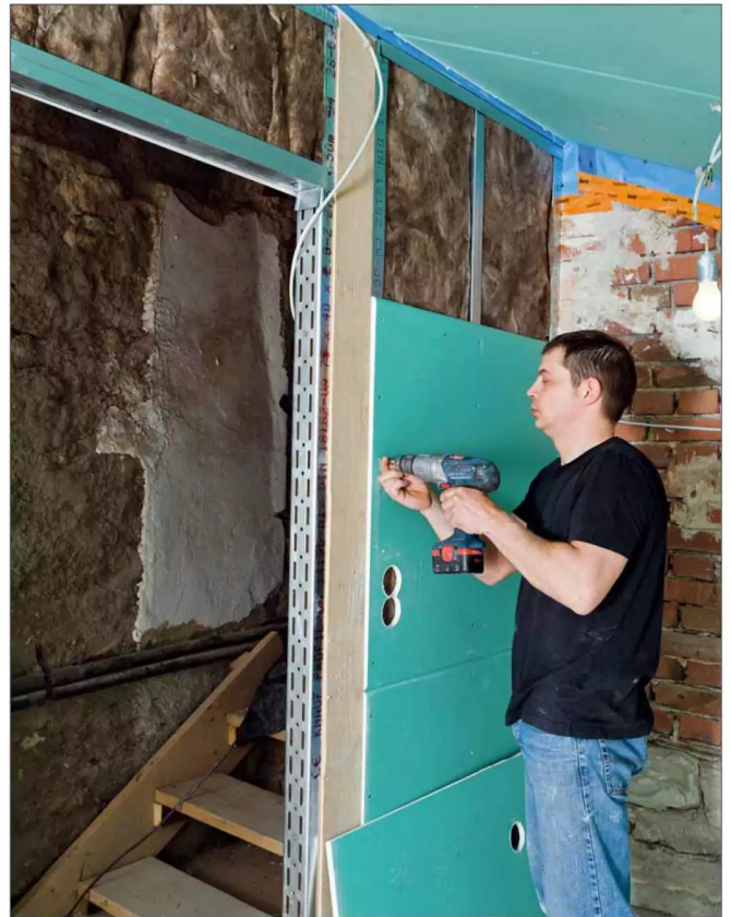
4 Je nach Plattenbreite und der Beplankungsrichtung (längs oder quer) ergeben sich verschiedene Achsabstände der Metallunterkonstruktion. Bei mehrlageriger Beplankung werden die einzelnen Plattenlagen mit versetzten Stößen gemäß dem Beplankungsschema montiert. Die Fugen der ersten Plattenlage sind hierbei auch zu verspachteln
