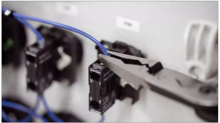
Halten oder Anklemmen von Einzeladern ist Standard
