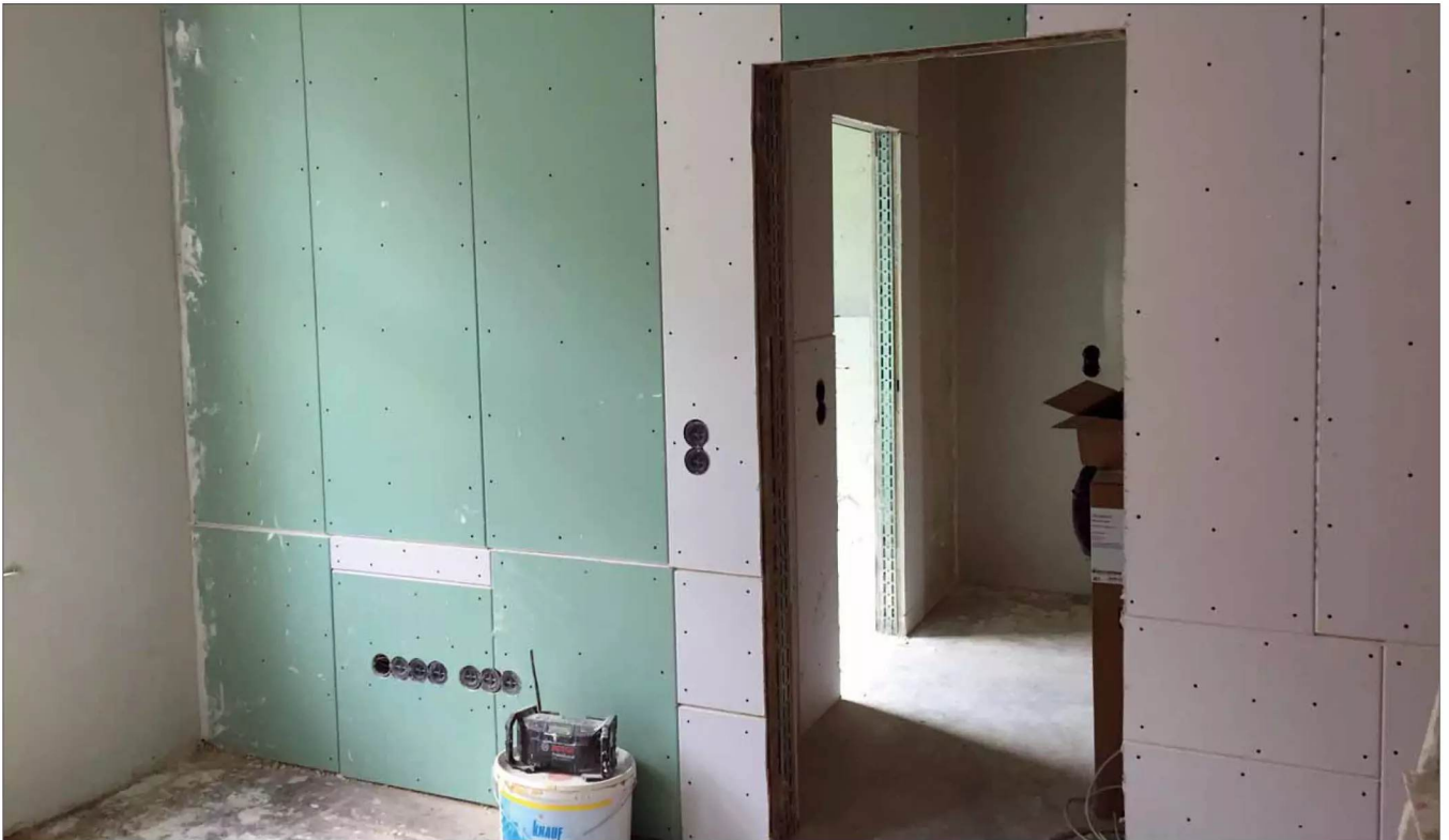
Die Verkleidung steht, aber die Flächen müssen noch verspachtelt werden. Gut sind die Schraublöcher an den Platten zu erkennen
