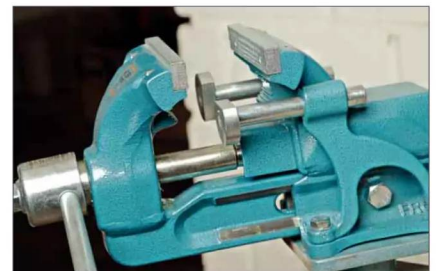
Einfach aber effektiv: Hier erkennt man prima das Funktionsprinzip der Auflagen. Werden sie nicht benötigt können sie einfach aus dem Spannungsbereich geschoben oder komplett herausgenommen werden
