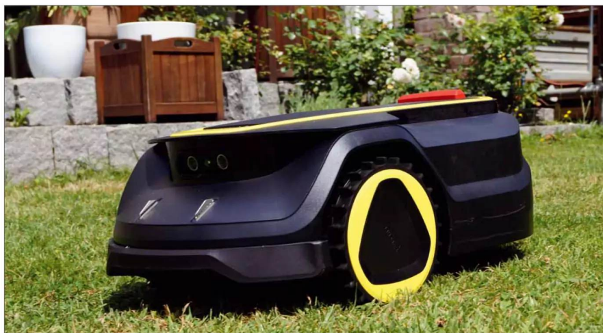
In der Vorderansicht sieht man die zwei Kameras und die Ladkontakte
