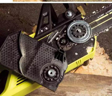
Zur Geräuschreduzierung soll die Dämpfung im Kettendeckel beitragen
