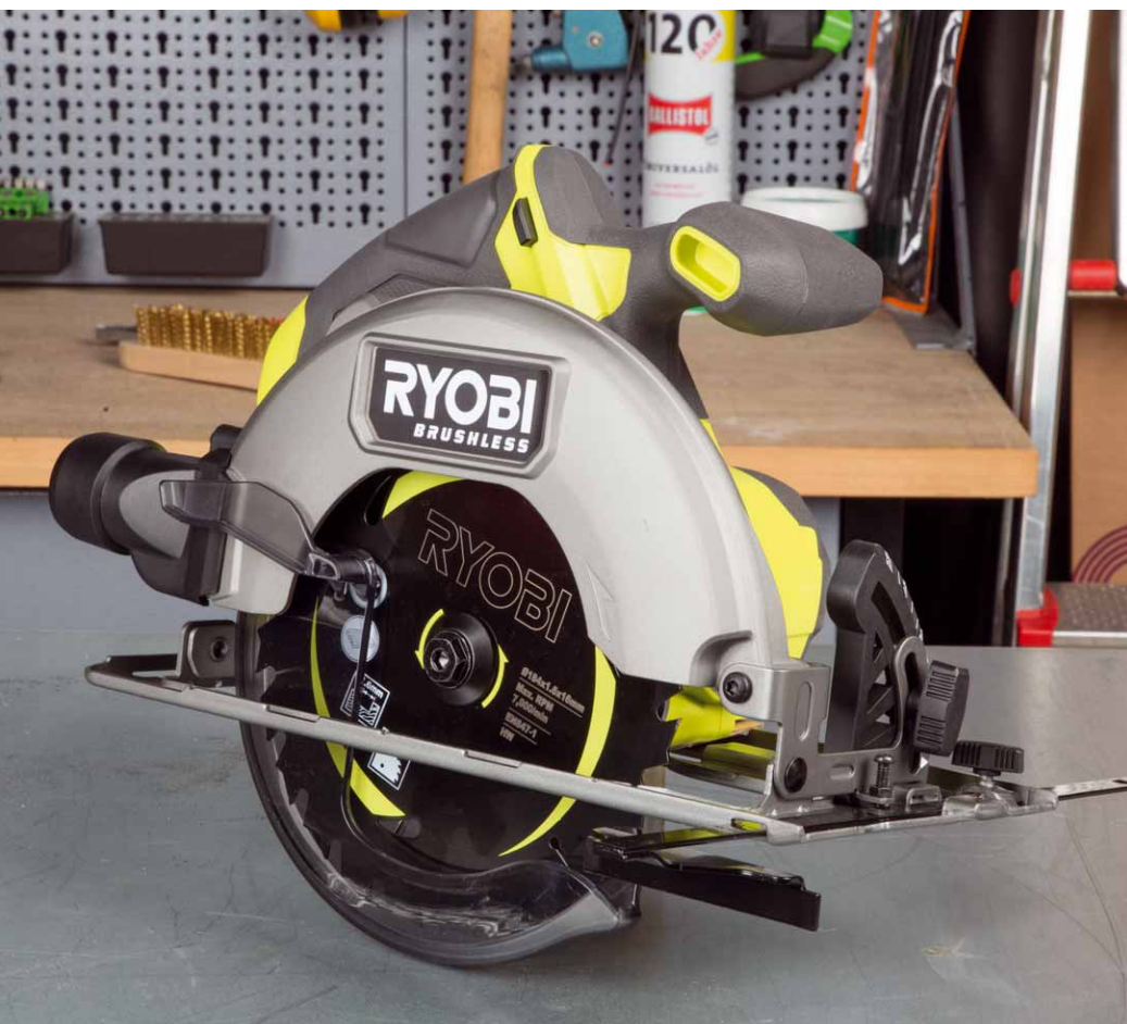
Der kleine Spoiler vor den Kühlschlitzen lenkt die Abluft direkt vor das Sägeblatt
