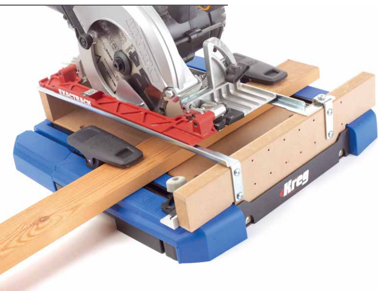
Das Tool KMA4100 macht aus einer Handkreissäge eine Kappstation
