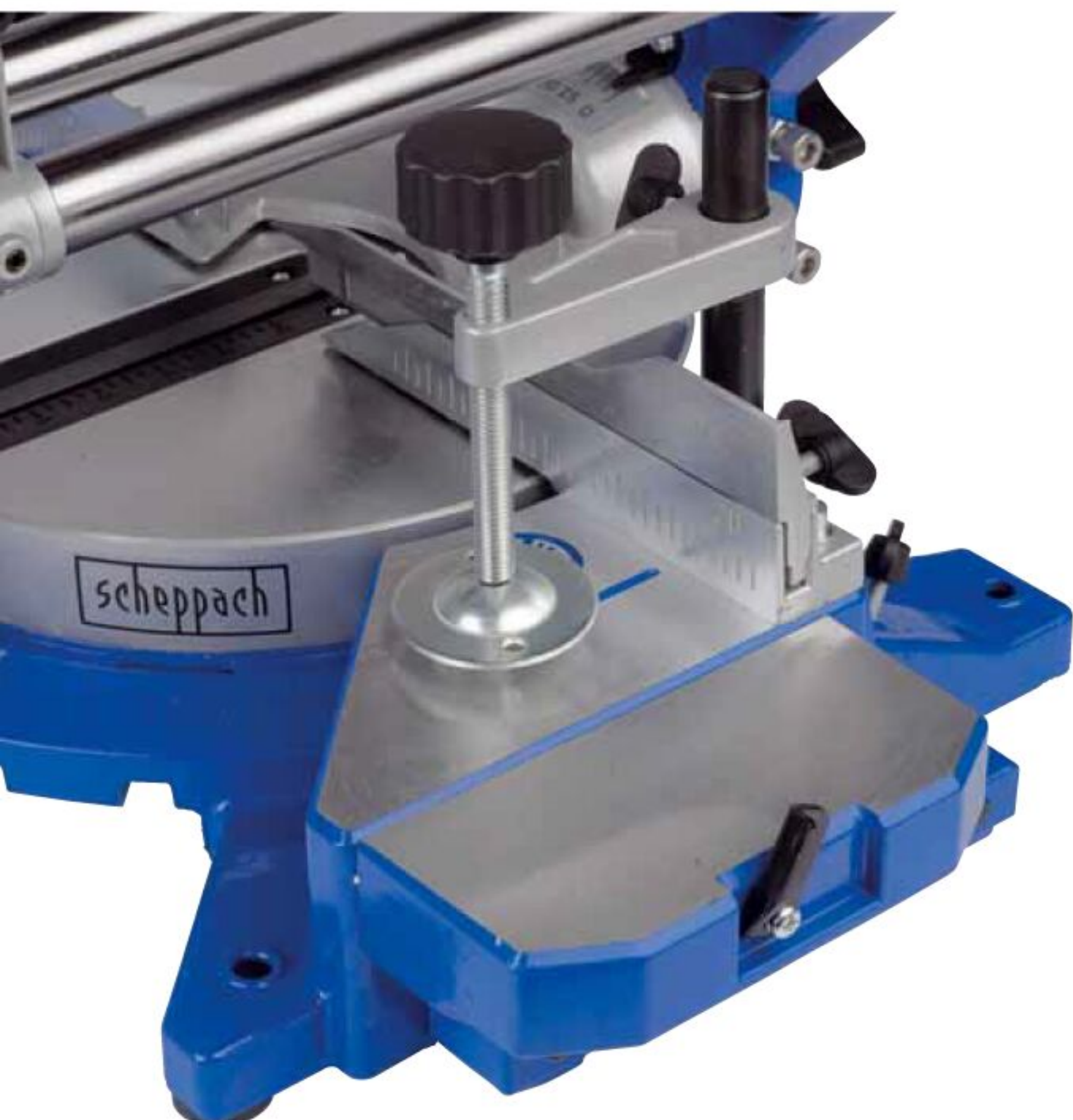
Der zweiteilige Niederhalter lässt sich schnell lösen und fest drehen
