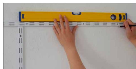
Mit Hilfe von Wasserwaage und „Zollstock“ werden die Montagepunkte für die zweite Schiene ermittelt
