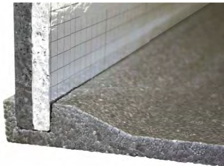
Die Komponenten werden nach dem Zuschnitt einfach zusammengesteckt
