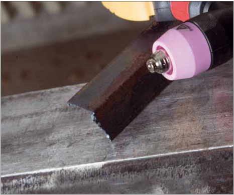
Wer mit einem Plasmabrenner gerade Schnitte machen möchte, braucht entweder viel Übung oder einen Anschlag an dem er den Brenner entlangführen kann
