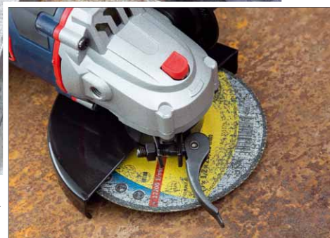
Um den Schnellverschluss so einzustellen, dass er den nötigen Halt am Maschinenhals findet, muss die Mutter an der Spannschraube eingestellt werden
