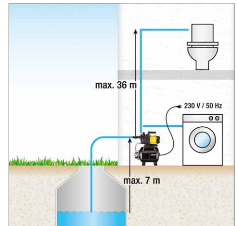
Dieses Diagramm zeigt den grundsätzlichen Aufbau einer Anlage zur Regenwassernutzung. Herstellerangaben zu Saug- bzw. Förderhöhe sind in solchen Diagrammen oft sehr großzügig angegeben
