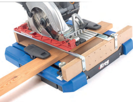
Der Werkstückhalter können auch kleine Werkstücke gut gesichert werden
