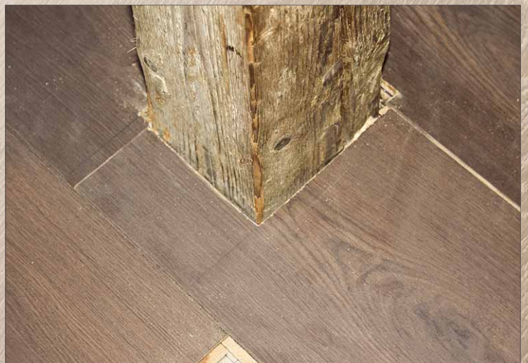
12 Die Stützbalken werden in den Boden eingepasst, auch hier sind die Fugenabstände einzuhalten
