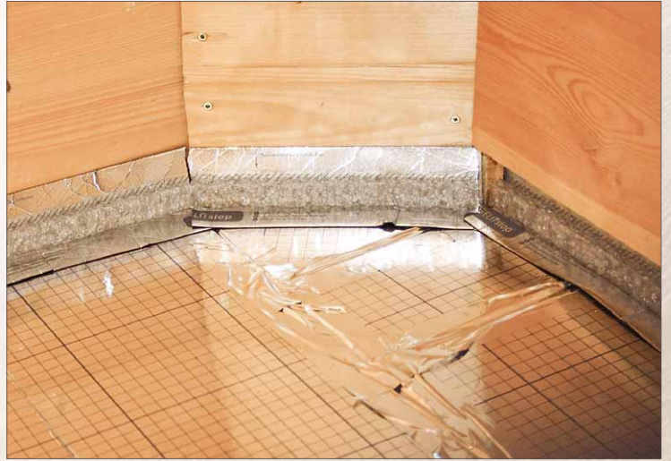
8 Wichtig bei der Verlegung ist, dass keine Ecken und Schrägen vergessen werden
