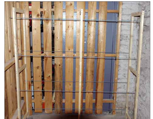
18 Sind alle Gewindestangen eingezogen und auf beiden Seiten mit Muttern und Scheiben gesichert, wird die mittlere Leiter an ihren Platz geschoben.
