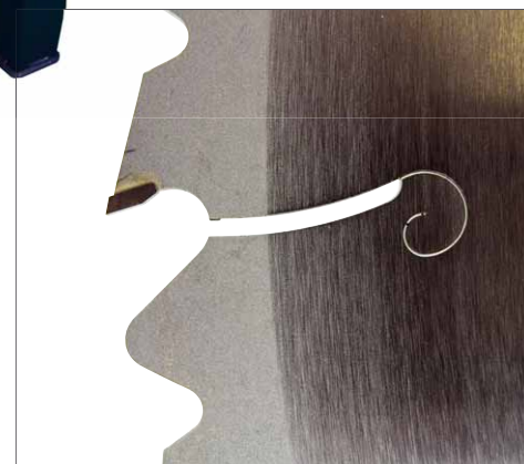
Die Einschnitte im Sägeblatt mit der nach unten auslaufenden Spirale dienen nicht der schönen Optik, sondern dem ruhigen Lauf. Die „Muster“ sorgen dafür, dass das Sägeblatt nicht in Schwingung geraten kann
