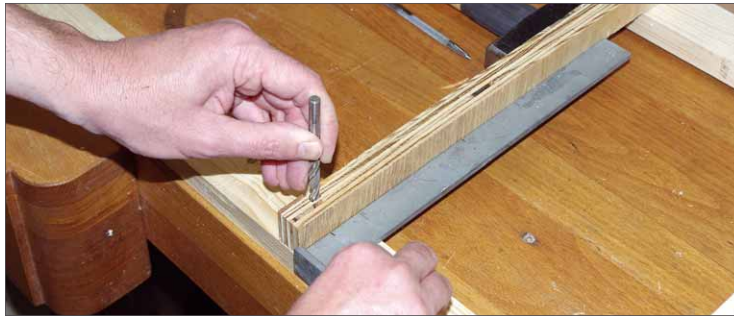
14 Die Positionen der Bohrungen für die Gewindestangen zeichnet man am besten mit einer Schablone an (einem Reststück Boden?). Die Schablone auf den Leitern dort positionieren, wo später ein Boden hin soll, rechtwinklig ausrichten und mit einem Bohrer die Mitte der Bohrung anstecken. Ggf. nochmal mit einer Spitze nachstechen
