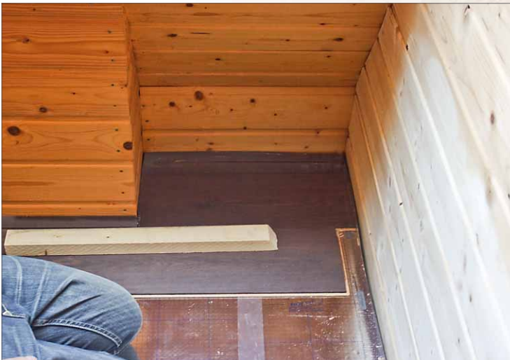
9 Nun können die ersten Reihen verlegt und eingepasst werden. Dabei kann es schon einmal am Ende knapp werden. In einem solchen Fall verwendet man zwei Paneele, die jeweils mindestens 50 cm lang sein sollten, um die Lücke zu schließen. Die 50 Zentimeter Paneellänge sind nötig, damit die Klickverbindung stabil wird.
