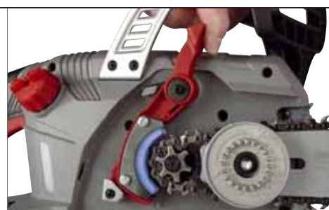
Mit dem integrierten Schleifstein wird die Kette in Sekunden geschärft
