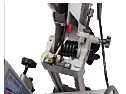
Hinter dem Schnittstellenlaser befindet sich die starke Feder, die den Maschinenkopf oben hält
