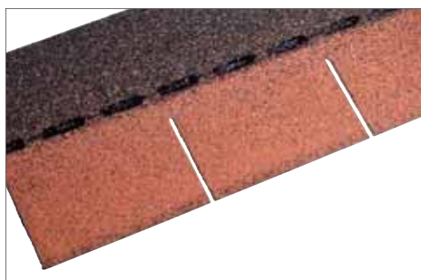
Für den unteren Dachabschluss wird der geschlitzte Schindelteil der Platten abgetrennt
