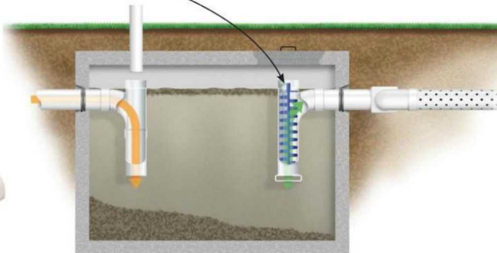
EFFLUENT FILTER
