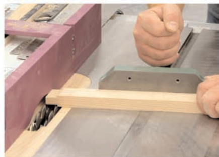
Angle fit rung tenons
