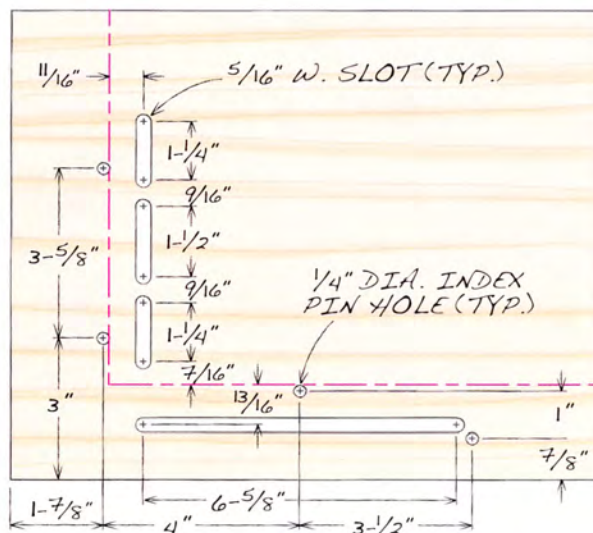
Fig. E Mortising Template
