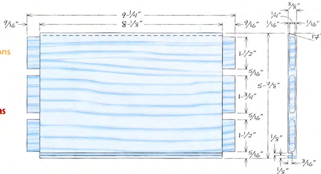
Fig. E Mortising Template
