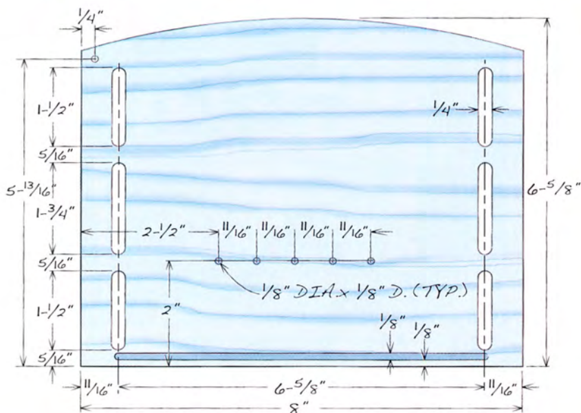
Fig. C End Dimensions
