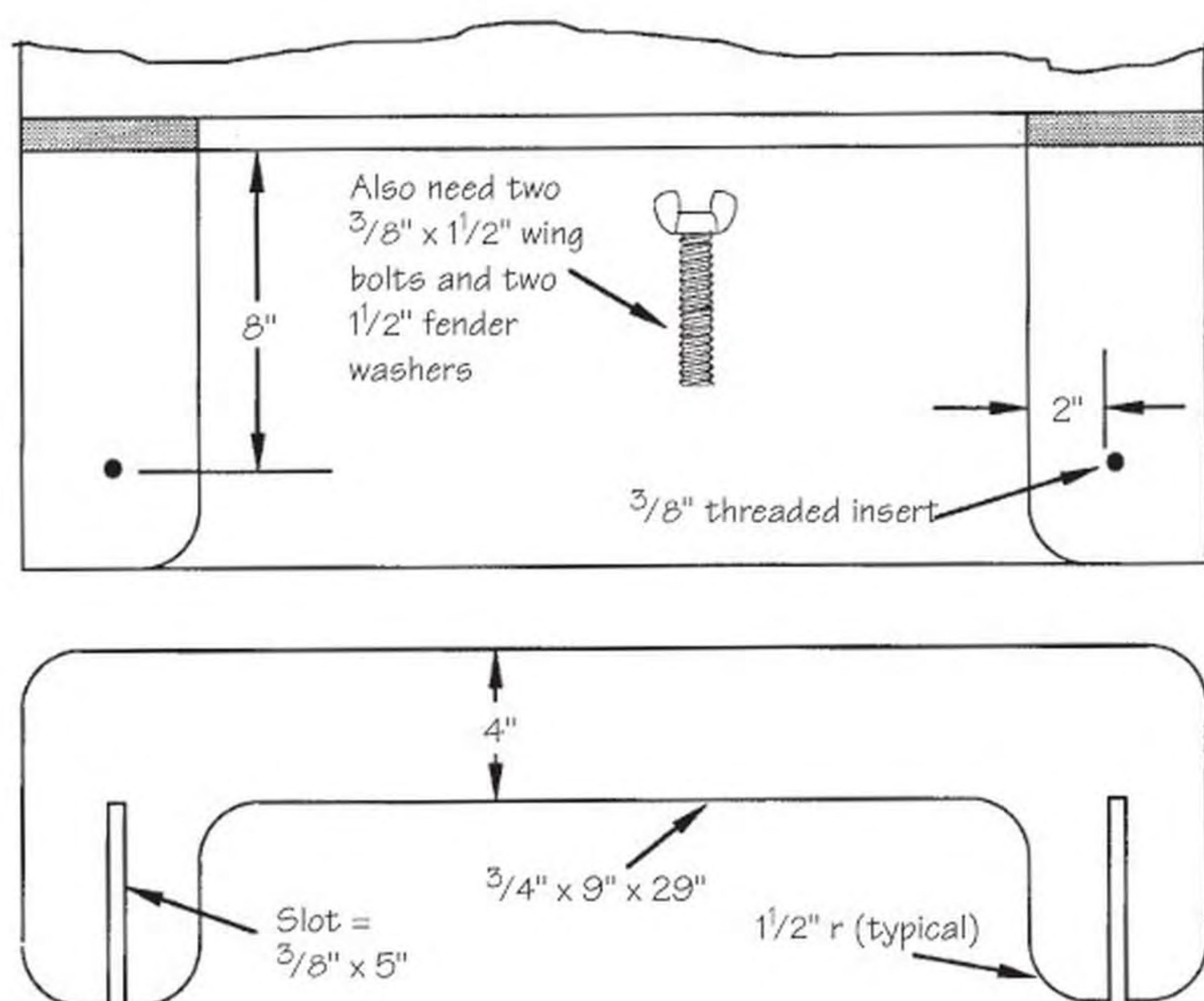
DIAGRAM 7 OPTIONAL HOLD-IN
