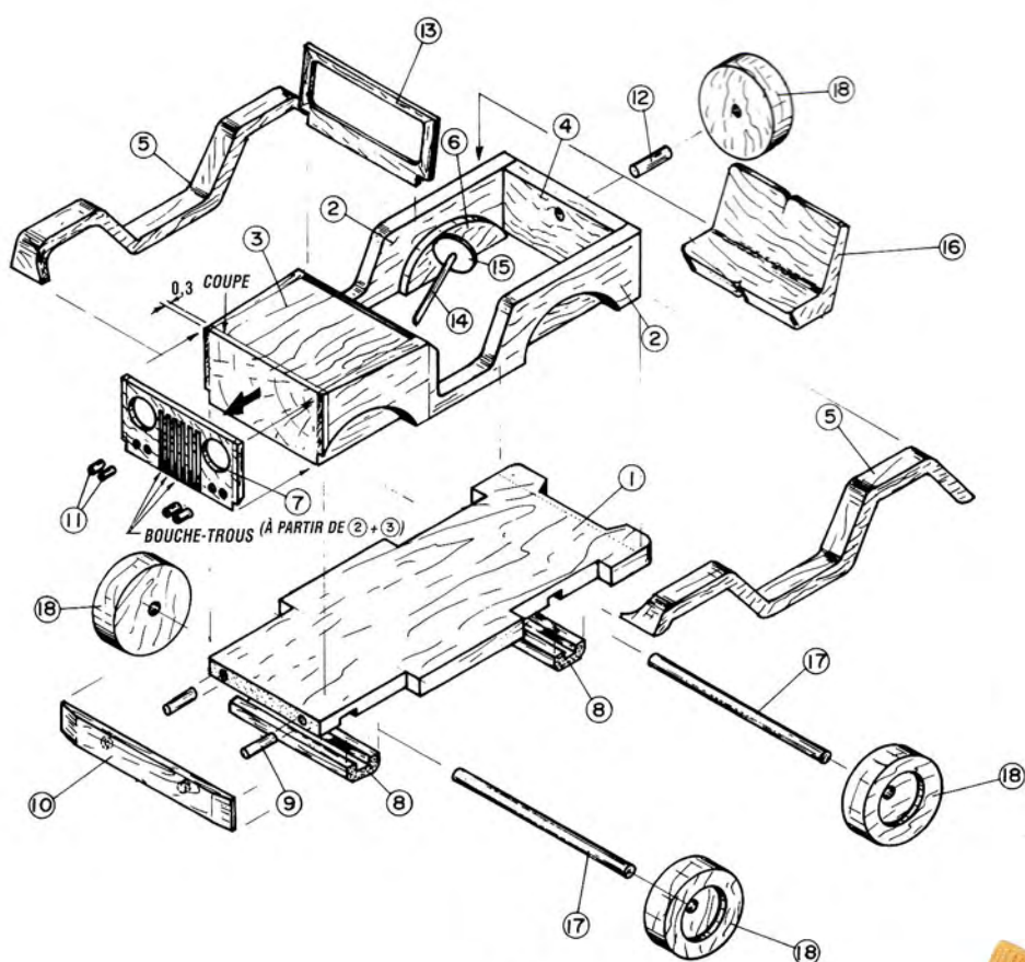
VUE ÉCLATÉE
