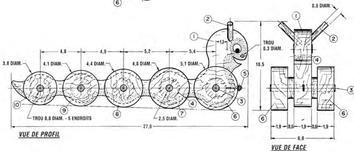
VUE ÉCLATÉE
