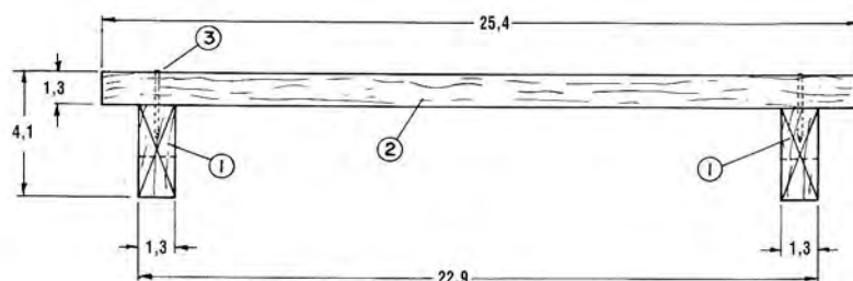
VUE LATÉRALE
