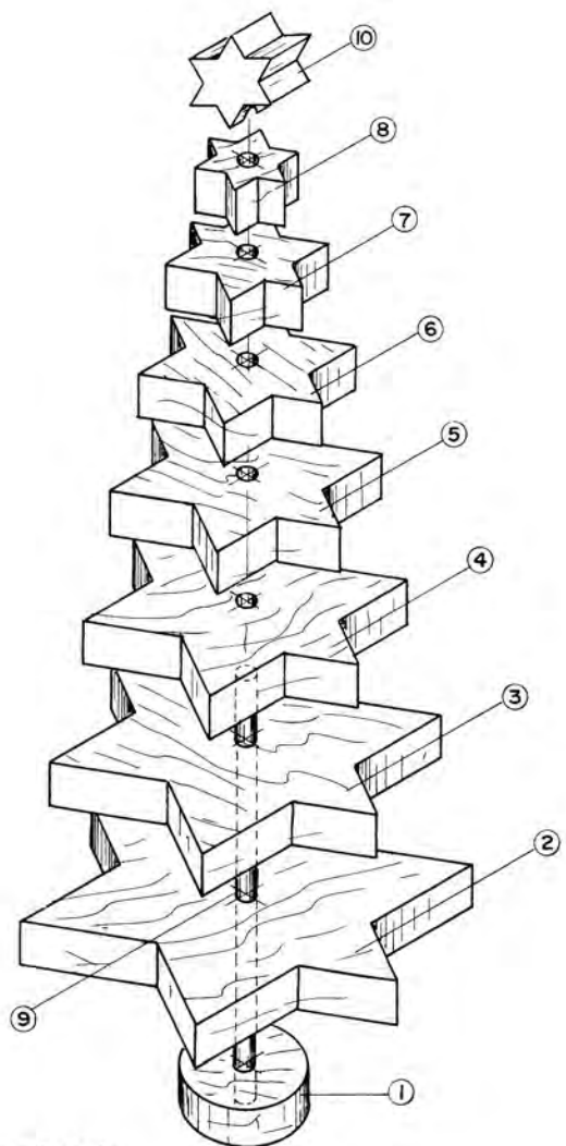
VUE ÉCLATÉE
